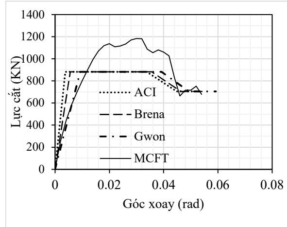
Hình 5. Mô hình dầm nối tính theo ASCE 41-13, Brena, Gwon và MCFT
