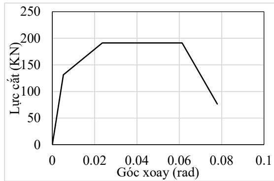
Hình 8. Dầm nối làm việc sau đàn hồi
